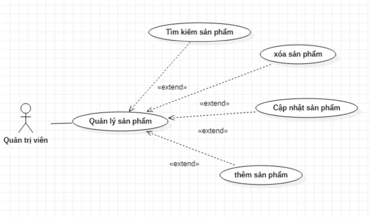
Hình 8: Use case quản lý sản phẩm
