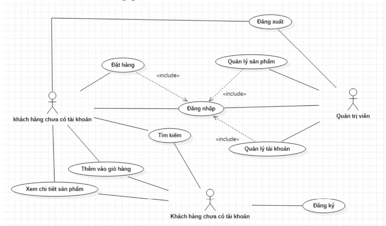
Hình 5: Sơ đồ use case tổng quát
