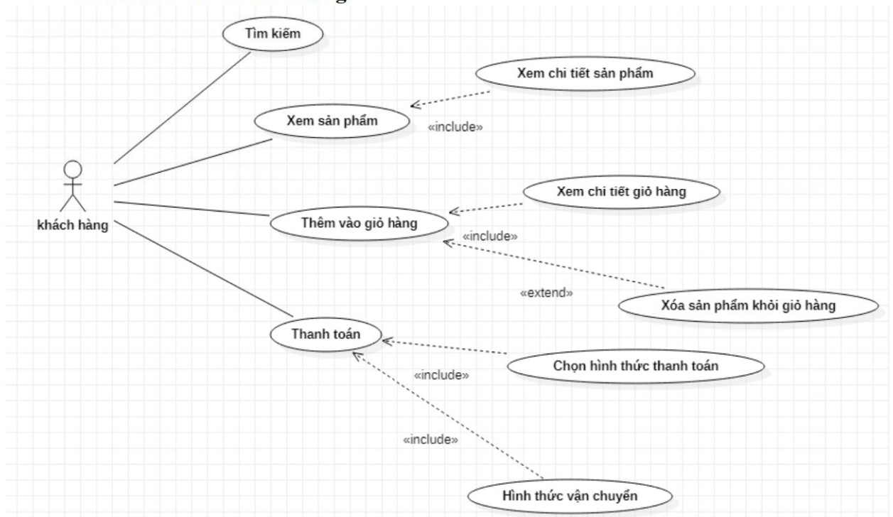
Hình 7: use case mua hàng
