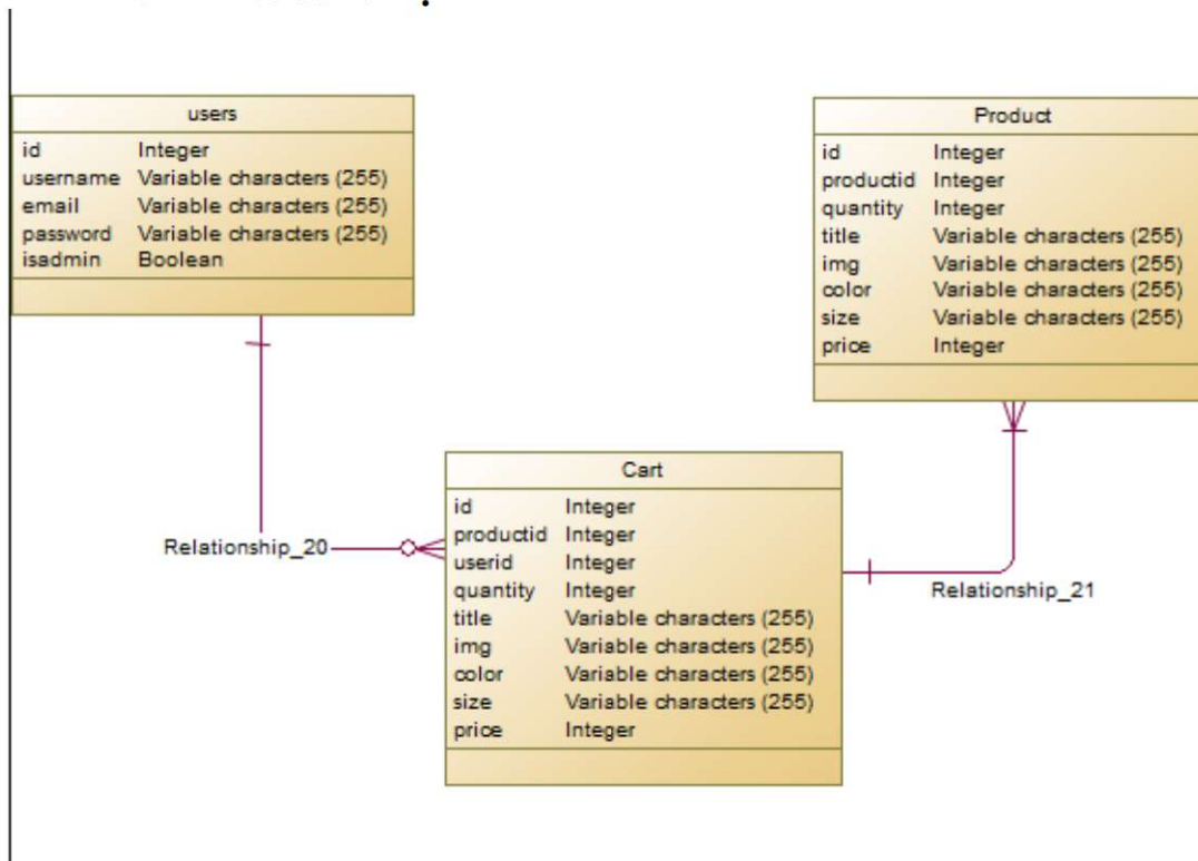
Hình 10: Mô hình CDM
